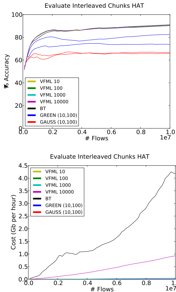
Fig. 1: Impact of the Numeric Estimator parameter
