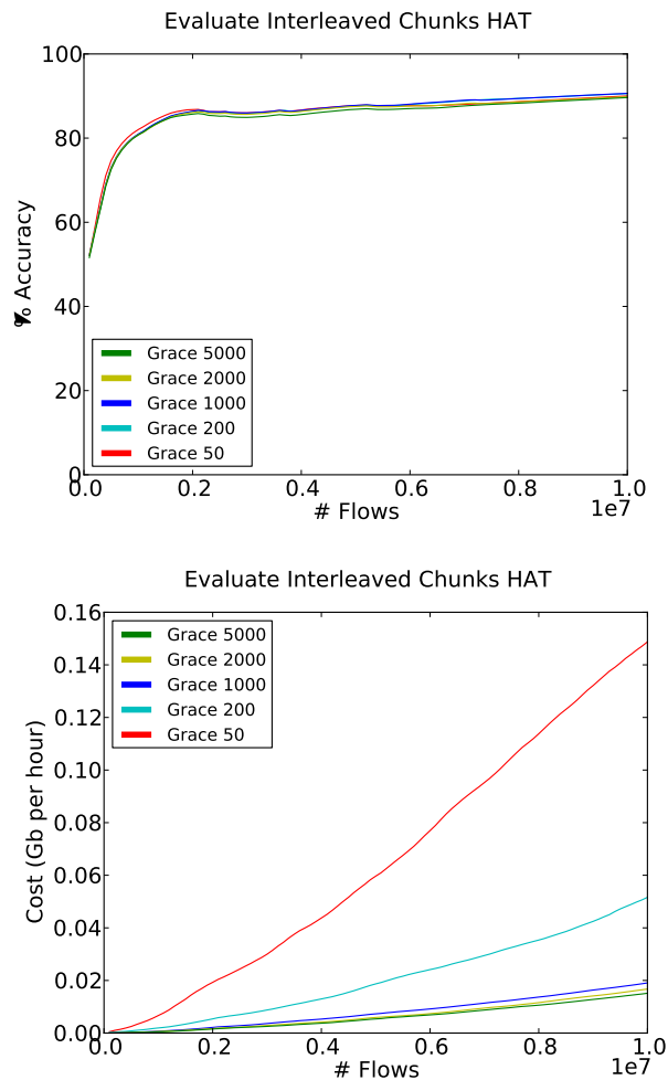
Fig. 2: Impact of the Grace Period parameter
